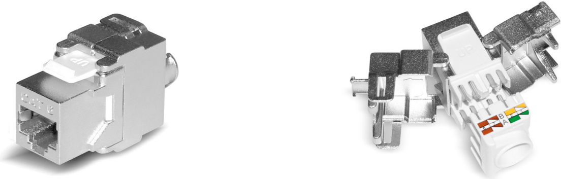
Module KS-T 5 1/8 toolless Cat.5e blindé
