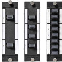
Plaques frontales FO-DCS-MTP, 3U/7HP, noir
